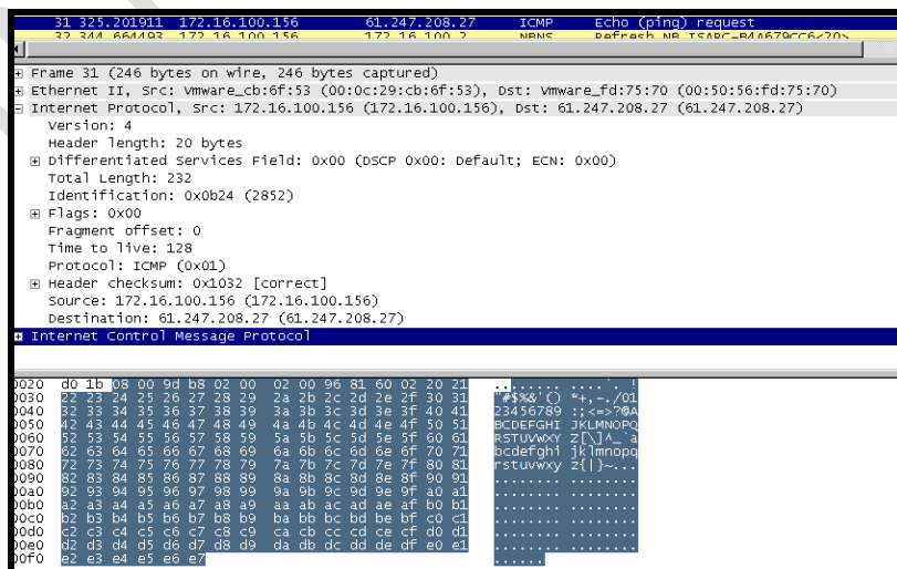
[ 그림 17. ICMP 공격 패킷 ]
