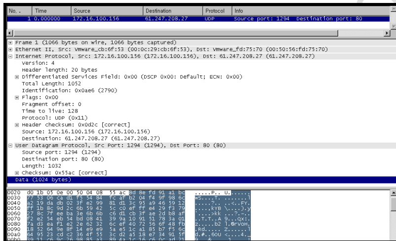
[ 그림 16. UDP 공격 패킷 ]
