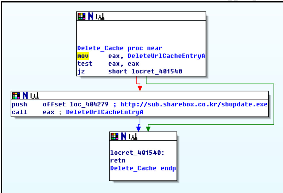
[ 그림 6. Url Cache 삭제 ]
