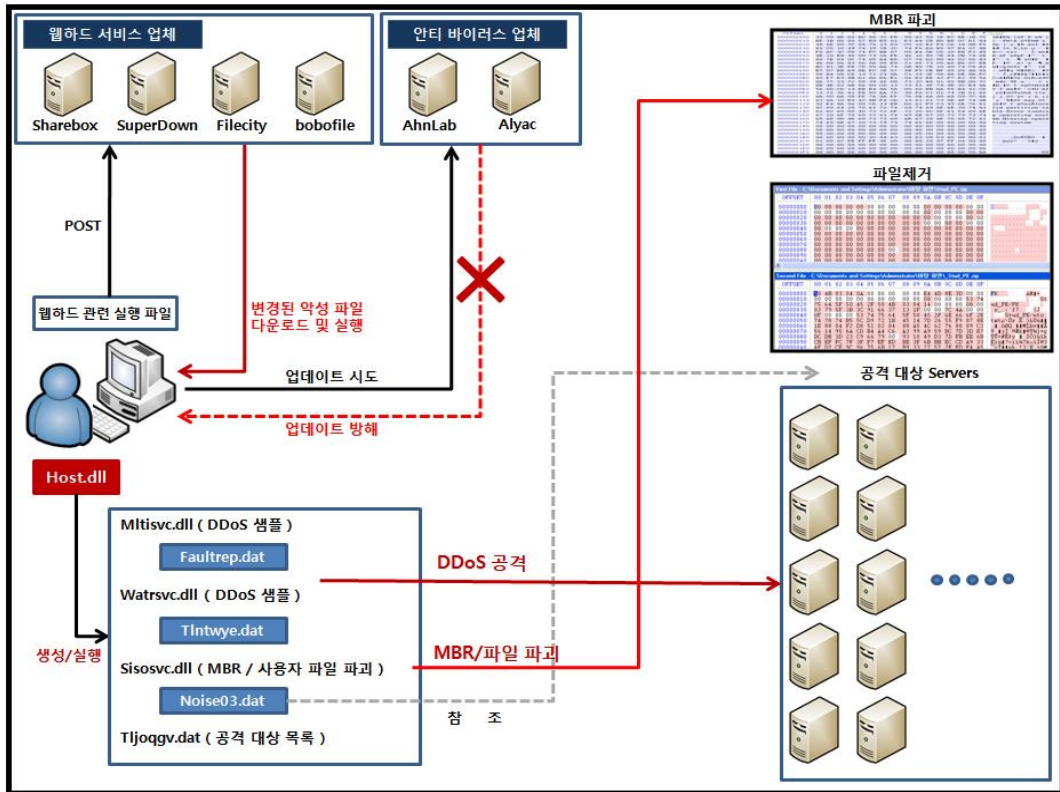
[ 그림 2. 파일간의 동작 과정 ]
