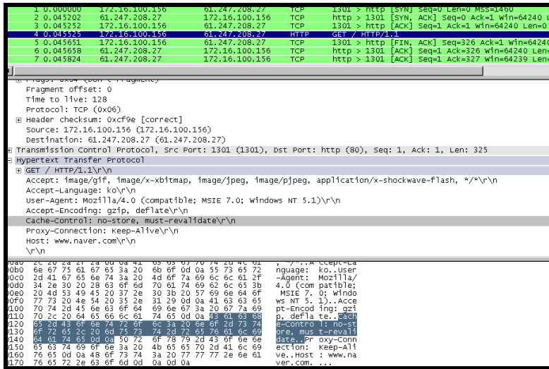
[ 그림 18. CC 공격 패킷 ]
