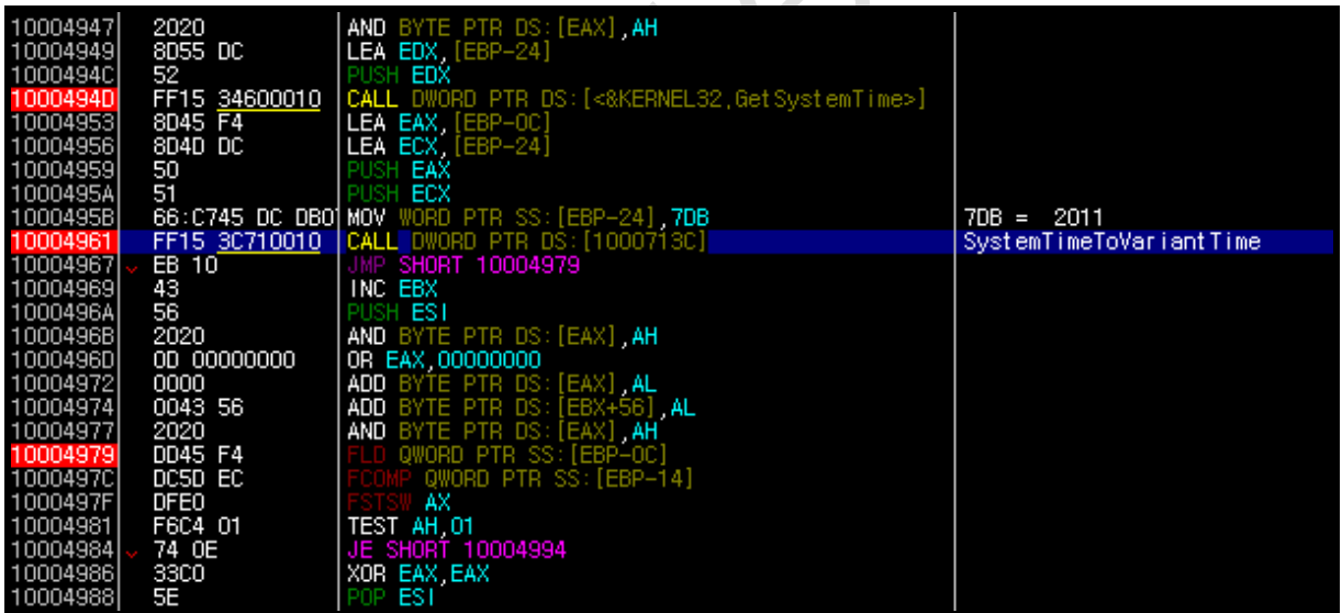
[ 그림 19. DDoS 공격 시간 관련 ]
