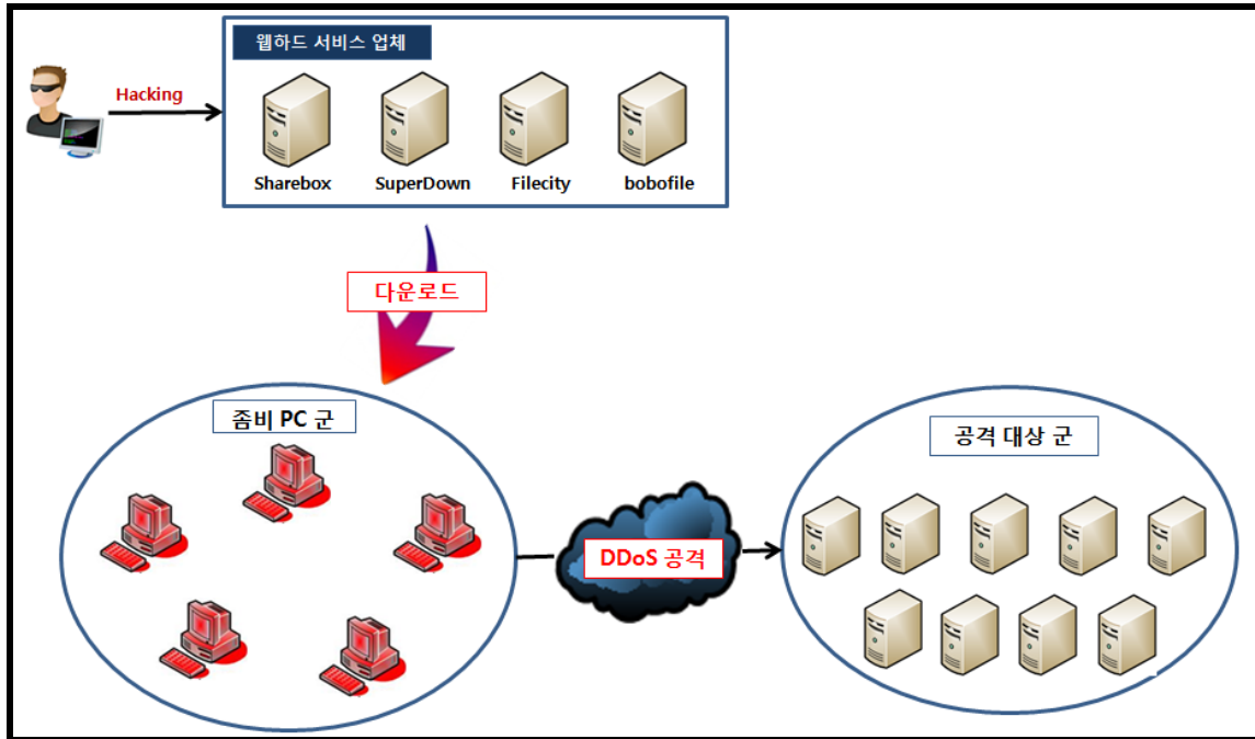
[ 그림 1. DDoS 전체 동작 시나리오 ]
