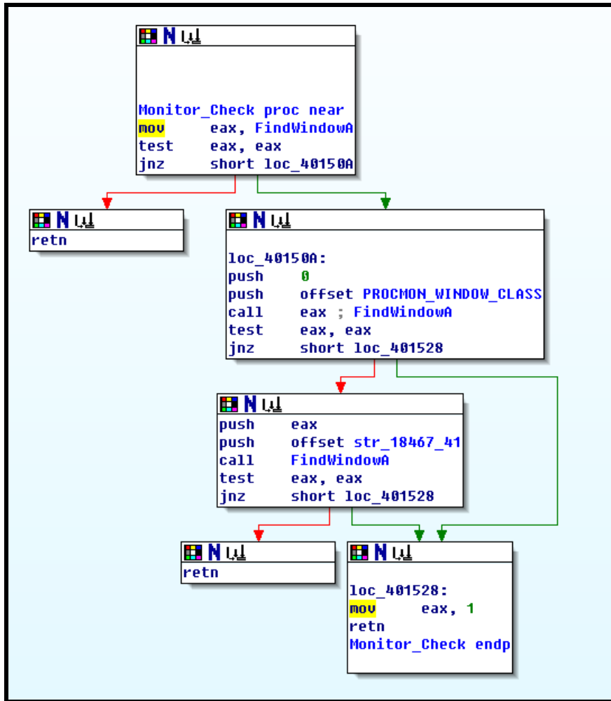
[ 그림 4. Monitor Tool 체크 ]
